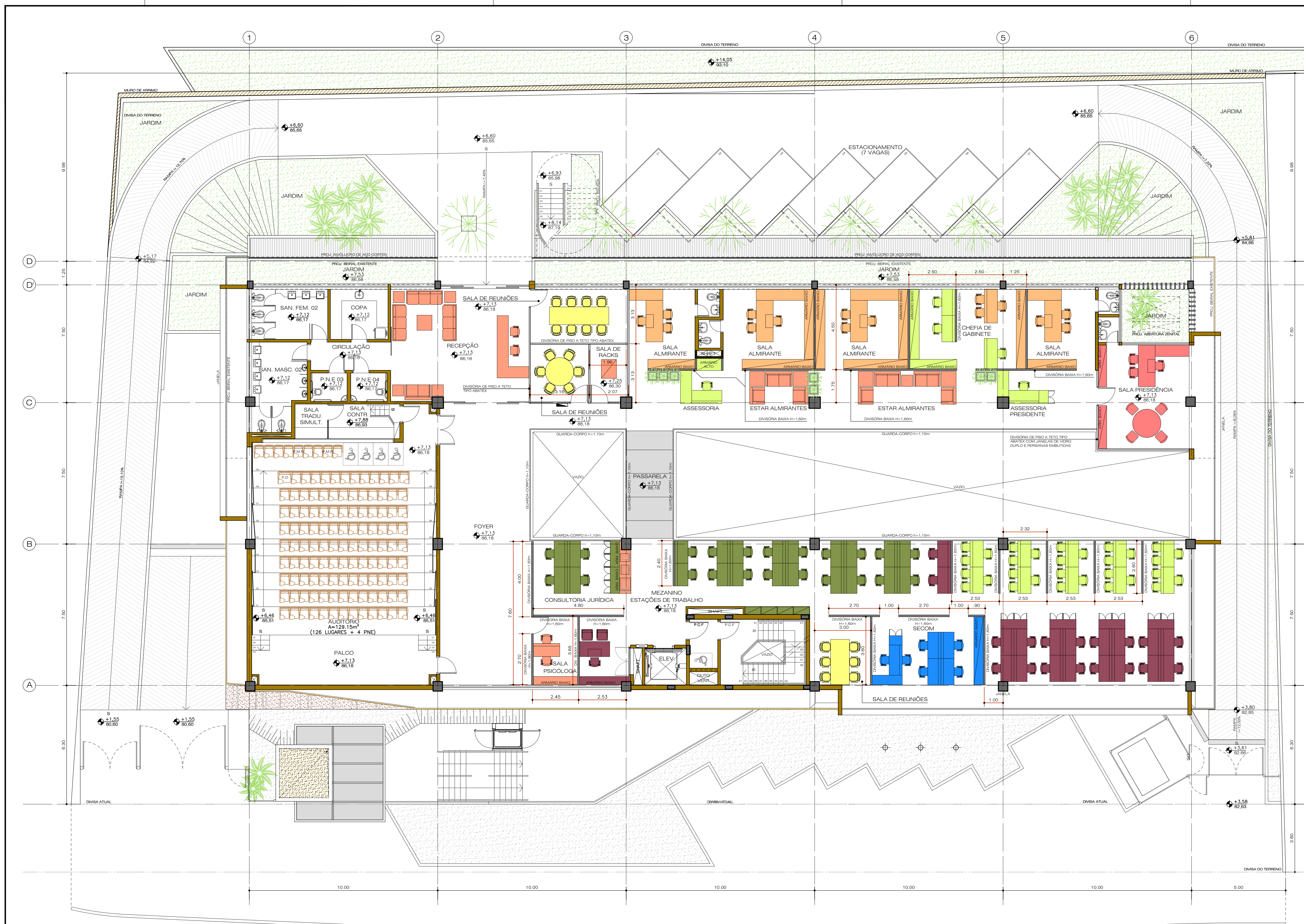
PLANTA MEZANINO - NÍVEL 86,18 = +7,13 ESC.: 1:100 0 1 5 10 ESCALA GRÁFICA
